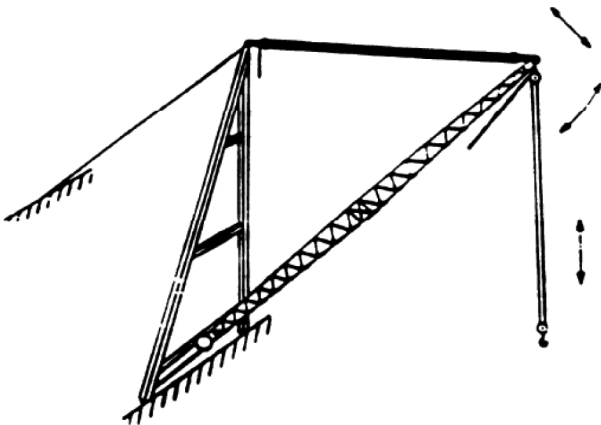
A-Frame Derrick
