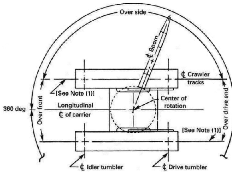
(d) Crawler Type Lower [Note(2)]
